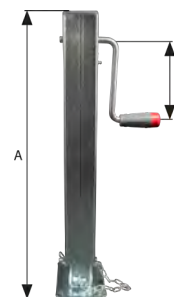
Schwerlast-Kurbelstütze 70 x 70 mm Vierkantrohr verzinkt
