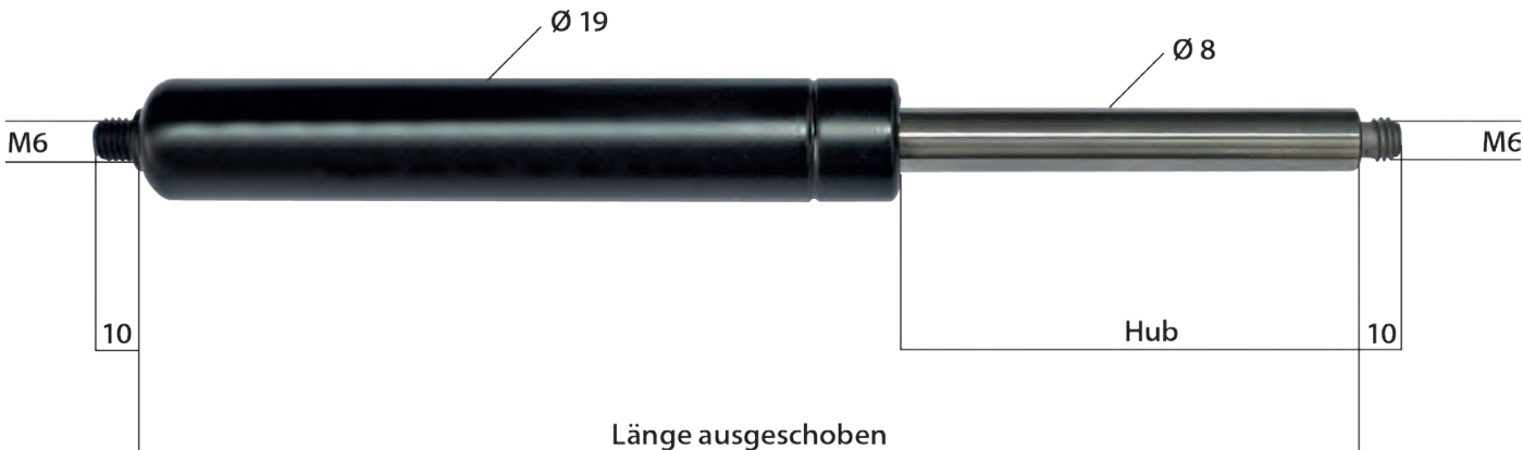
Gasfedern 08 / 19 100 N - 300 N
