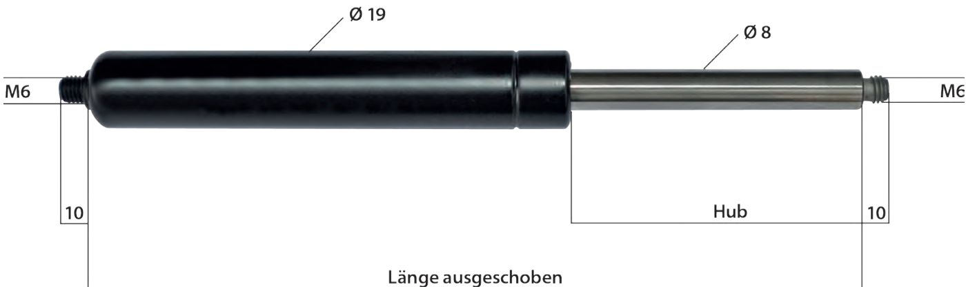
Gasfedern 08 / 19 350 N - 500 N
