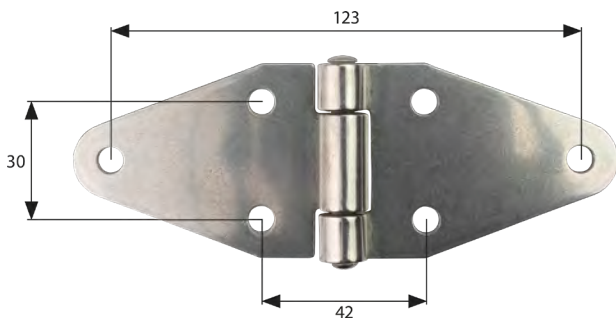
Faltscharnier, Nirosa Edelstahl, gerollt Bohrungs-Ø 6,5 mm je Seite
