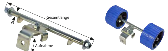
Steigbügel für Doppel-Kielrolle, regulierbar verzinkt
