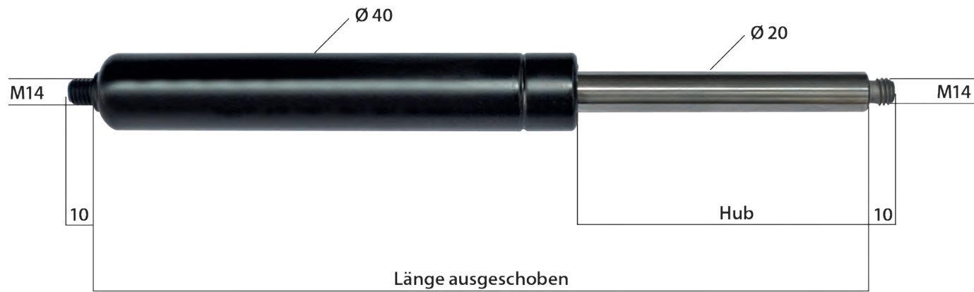
Gasfedern 20 / 40 3000 N - 5000 N
