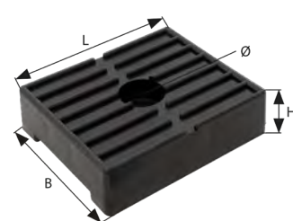
Bootsauflage Gummi
