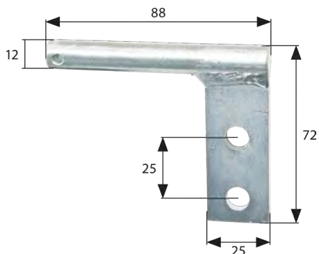
Scharnierlager für Auwärter Anhänger M + GL Bohrungs-Ø 3,8 / 9,5 mm
