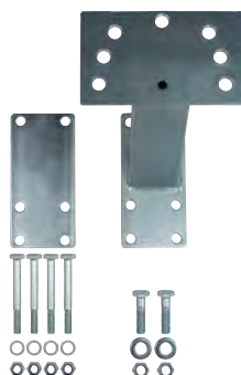
Ersatzradhalter zum Klemmen, universal
