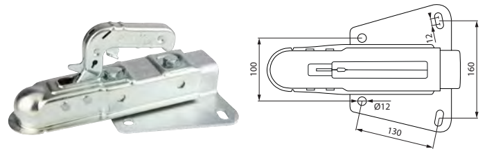
Kugelkupplung AL-KO AK 7 Plus - 75 V für V-Deichsel
