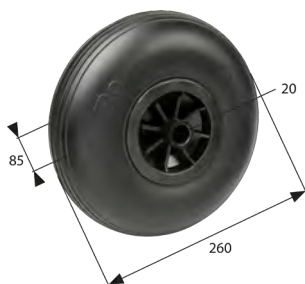
PU-Rad mit Kunststofffelge, Tragfähigkeit 100 kg Füllung aus PU-Schaum
