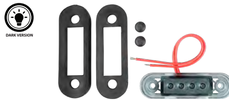
Begrenzungsleuchte LED, rot, DARK 12 - 36 V, Kabellänge 150 mm Maße (mm): 84,2 x 27,7 x 12,8
