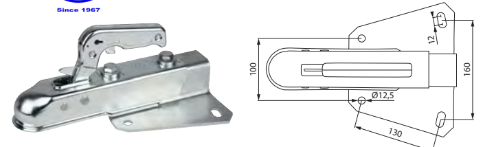
Kugelkupplung SPP DV-01.750 für V-Deichsel
