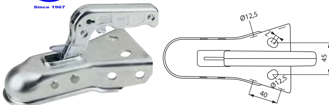
Kugelkupplung SPP ZSK-750K für V-Deichsel
