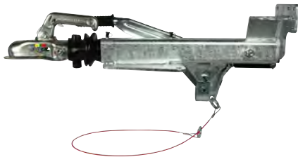
Auflaufeinrichtung WAP mit Stützradkonsole hinten
