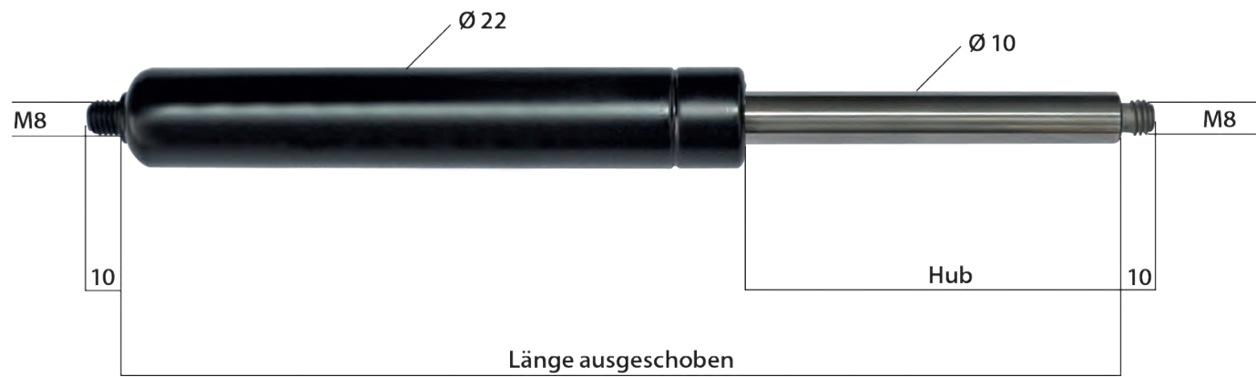
Gasfedern 10 / 22 550 N - 900 N
