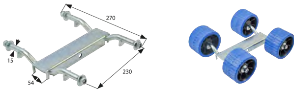
Steigbügel für 4-fach-Kielrolle, verzinkt
