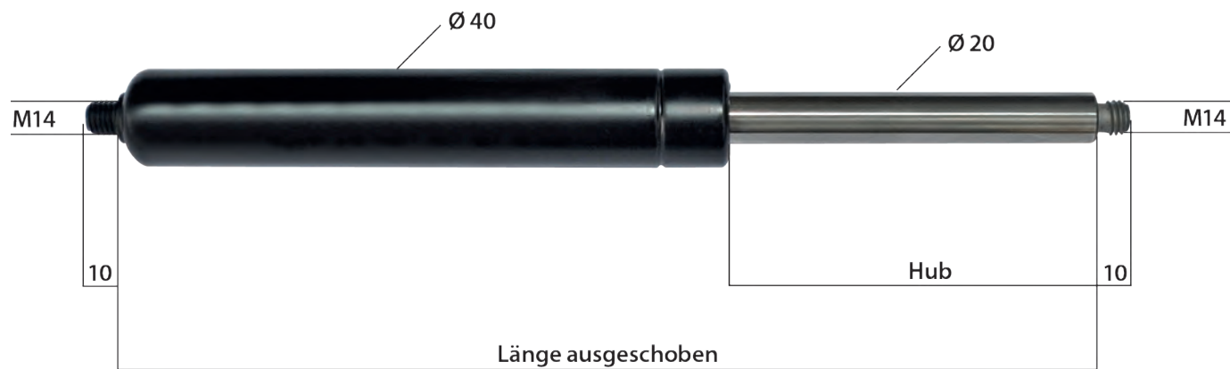
Gasfedern 20 / 40 500 N - 2500 N
