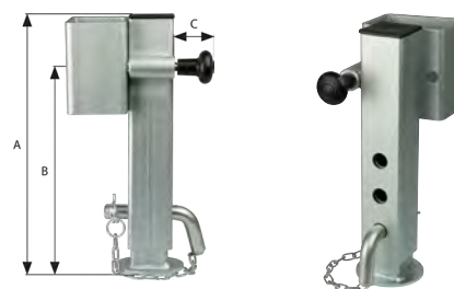
Stützfuß, klappbar, 60 x 60 mm Typ TL60, mit Teller Ø 90 mm Vierkantrohr verzinkt
