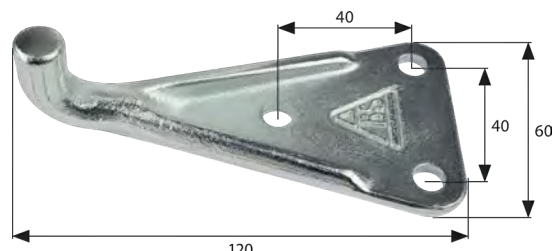
Gegenhalter für Excenterverschluss zum Anschrauben, verzinkt Bohrungs-Ø 8,5 mm, Haken-Ø 13 mm
