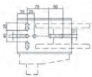
Handseilwinde, Typ SSW 900/1 mit Abrollautomatik mit Trommelfreilauf ohne Seil Kurbel abnehmbar
