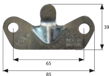
Gegenhalter für Spannverschluss zum Anschrauben, verzinkt Bohrungs-Ø 9,0 mm, Stärke 4 mm
