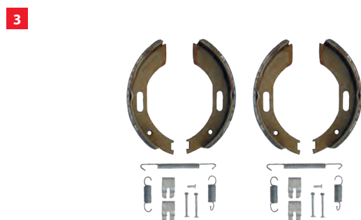
Bremsbackensatz BPW, 200 x 50 Satz für eine Achse, mit Federnsatz
