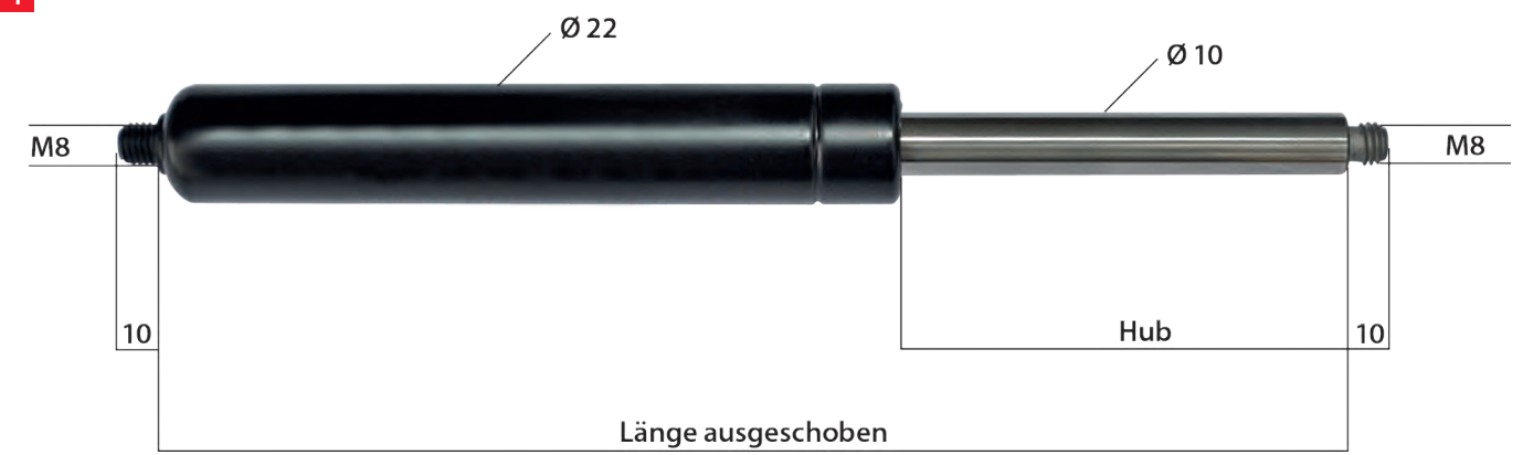
Gasfedern 10 / 22 150 N - 500 N
