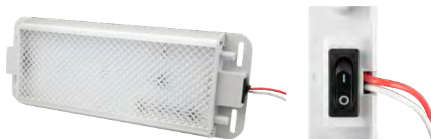
Innenleuchte LED mit Schalter Kabellänge 400 mm, 7,7 W Zertifizierung CE, IP65
