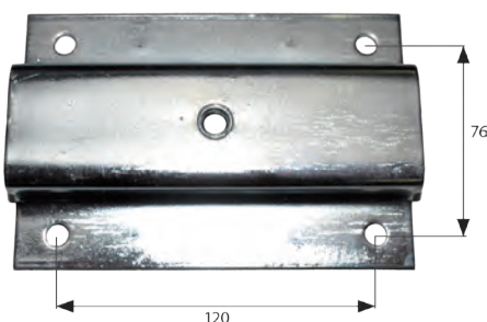
Rungenhalter Stahlblech, mit eingesch. Mutter M10, Bohrungs-Ø 9 mm für Rungen 20 x 40 mm (Bereich der Mutter 13 x 40 mm)
