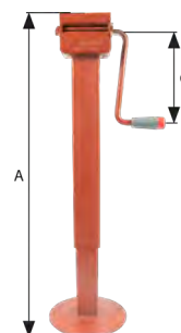
Kurbelstütze 70 x 70 mm Vierkantrohr mit senkrechter Kurbel gründiert
